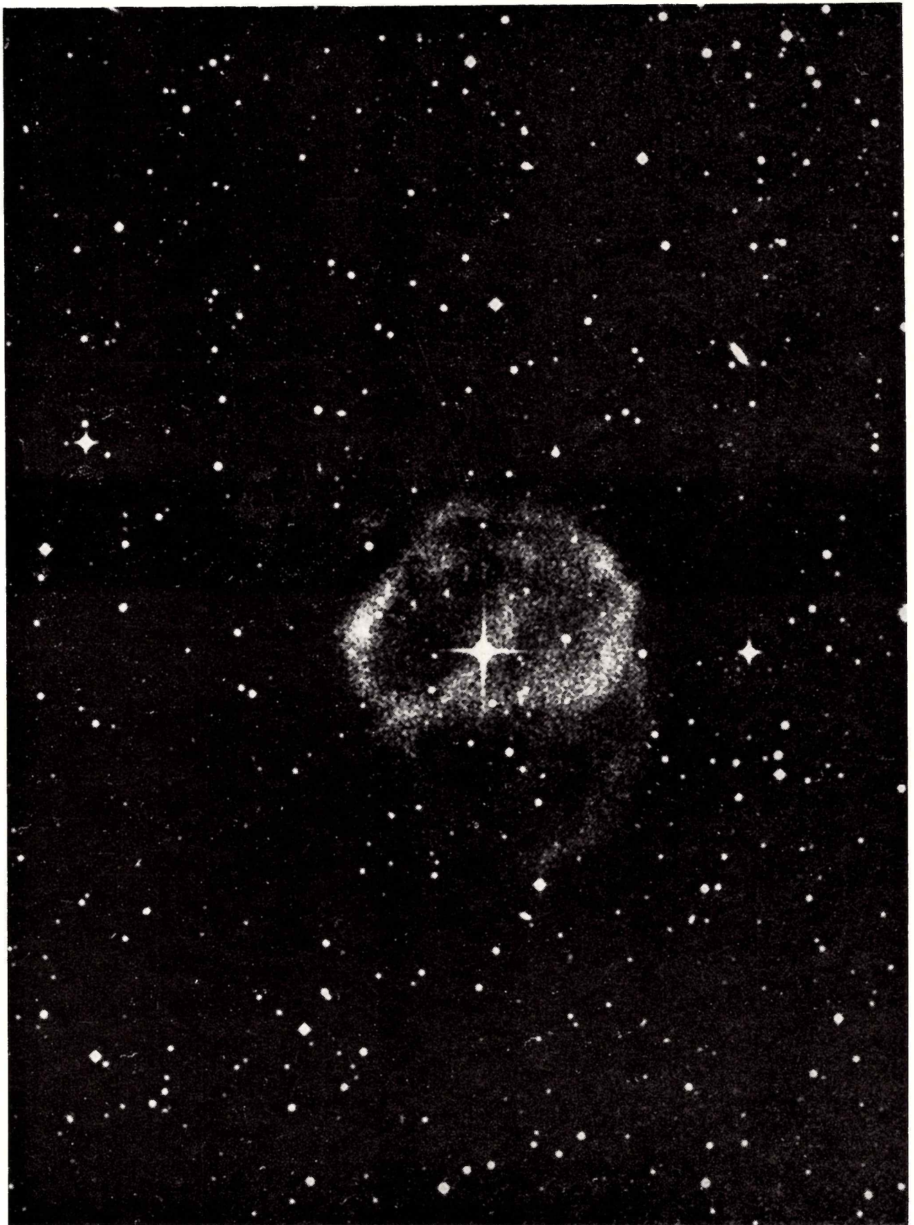
Planetárnu hmlovinu Abell 36 objavil Abell v roku 1955. Rozmery 478 \times 281 oblúkových sekúnd a celková jasnosť asi 13^m pri vzdialenosti zhruba 1400 svetelných rokov radia túto hmlovinu medzi veľké a teda aj staré objekty svojho druhu. V skutočnosti má hmlovina priemer asi 3 svetelné roky a štúdium jej zaujímavej štruktúry nám môže veľa napovedať o procesoch, ktoré sa odohrali na začiatku jej expanzie.
