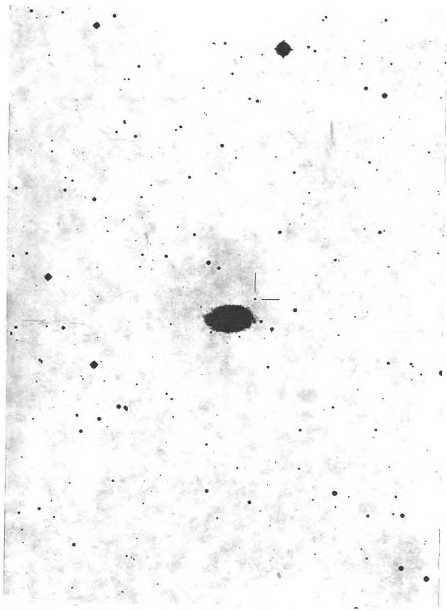
Stejná oblast jako na 2. str. obálky (okolí NGC 4753), reprodukována z fotografie č. 1578 Palomarského atlasu s označenou hvězdou v těsné blízkosti místa, kde byla objevena supernova. — Na čtvrté str. obálky je kulová hvězdokupa M 13 v souhvězdí Herkula, exponovaná v noci 9./10. VIII. 1962 Schmidovou komorou v Tautenburku. Expozice 7 min. se žlutým filtrem GG 13 na desku Agfa-Astro-Spezial.
