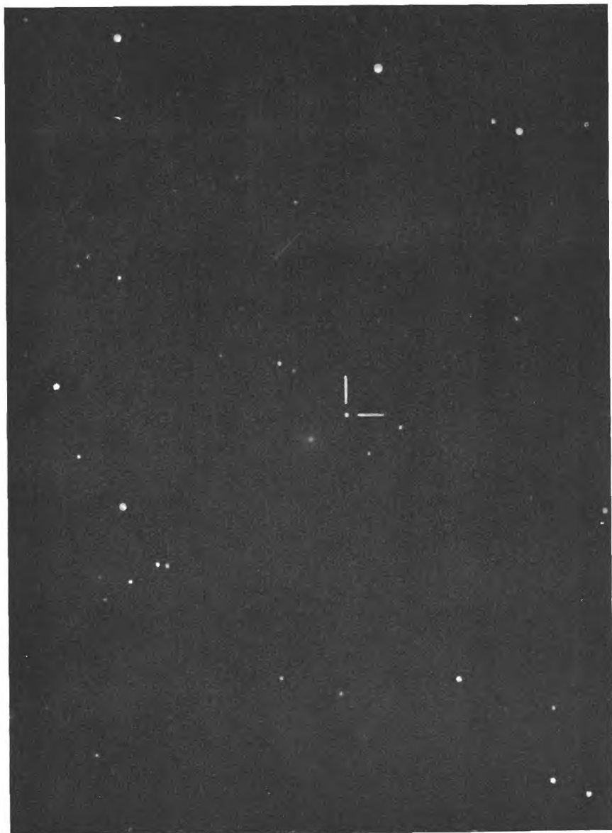
Fotografie okolí NGC 4753 s označenou supernovou, získaná na Skalnatém Plese dne 25. VI. 1965 reflektorem \varnothing 60 cm. Nejjasnější hvězda v horní části snímku (severně od supernovy) je BD -0^{\circ}2622 (9 m pg). K článku na straně 236 (foto M. Antal). — Na první str. obálky je spirálová galaxie M 51 v souhvězdí Honičích psů. Snímek Schmidovou komorou 200cm universálního reflektoru observatoře v Tautenburku dne 18. II. 1961 (expozice 60 min. na desku Agfa-Astro-Spezial).
