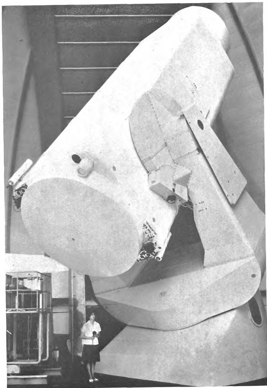
Dvoumetrový univerzální zrcadlový dalekohled observatoře K. Schwarzschilda v Tautenburku. (Snímek hvězdárny v Tautenburku.)
