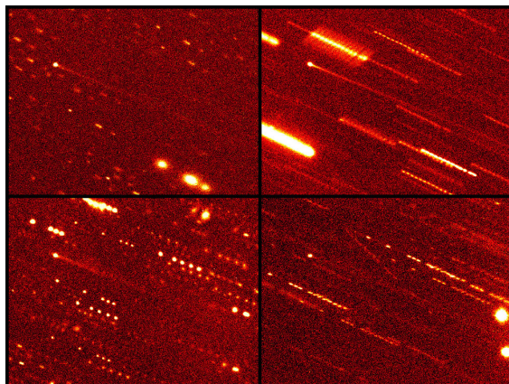
Obr. 3 — Snímky komety 133P/Elst–Pizarro pořízené během druhého období aktivity, 19. srpna, 7. září, 5.–7. listopadu a 27. prosince 2010, pomocí 2,2 m teleskopu University of Hawaii na observatoři Mauna Kea a CCD kamery Tektronix 2048×2048 pixelů (rozlišení 0,219"/pxl).
