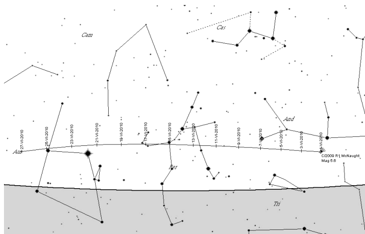
Obr. 7 — Vyhledávací mapka pro kometu C/2009 R1 McNaught.
