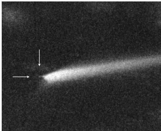
Obr. 2 — Snímek komety P/2010 A2 (LINEAR), který pořídili James Annis (Fermilab), Marcelle Soares-Santos (FermiLab a University of Sao Paulo) a David Jewitt (UCLA) 11. ledna 2010 pomocí 3,5 m dalekohledu WYNN. Bodové jádro je vyznačeno šipkami.
