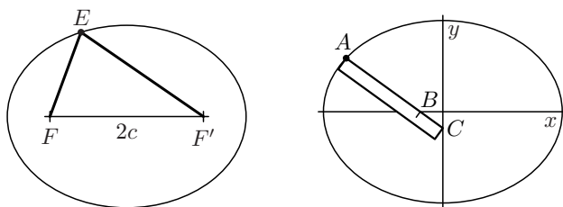
Obr. 7 — Dvě možnosti vytyčení elipsy: (a) pomocí napnutého lanka o délce 2a , (b) pomocí tyče o délce a .
