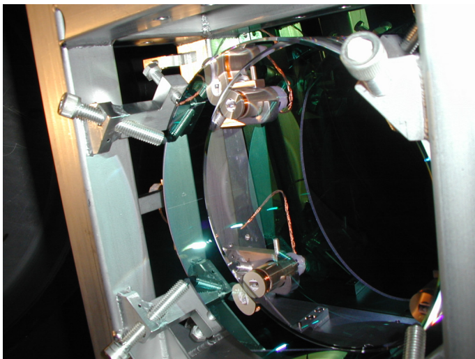
Obr. 14 — Jedno ze zrcadel interferometru LIGO. Převzato z [2].
