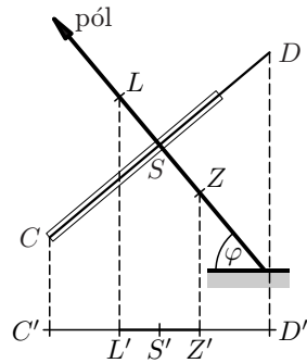
Obr. 5 — Průmět roviny rovníku do vodorovné roviny, pohled od východu.
