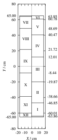
Obr. 8 — Náskres středové desky s datovou úsečkou pro analematické hodiny v Bohdanči.
