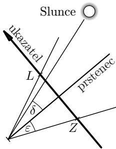
Obr. 4 — Situace v rovině kolmé k rovníku, která prochází sluncem a ukazatelem.
