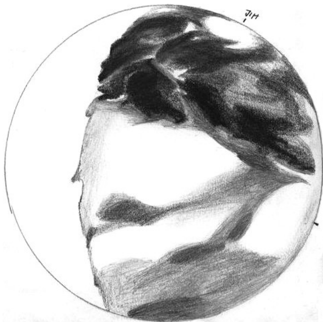
Obr. 18 — Mars 30. srpna 2005, 4 h 9 min až 4 h 21 min UT; přístroj: reflektor 0,25 m, f/5 ; zvětšení: 66krát; místo: Seč, Ústupky, pláž; podmínky: 8; teplota: 14 °C.
