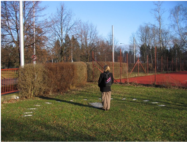
Obr. 11 — Analematické hodiny u Gymnázia Boženy Němcové, na Pospíšilově třídě v Hradci Králové. Středová deska těchto hodin je záměrně vyrobena kratší a nezahrnuje zimní měsíce, kdy hodiny obvykle nejsou využívány. Jejich konstruktérem je Jan Veselý a studenti gymnázia.
