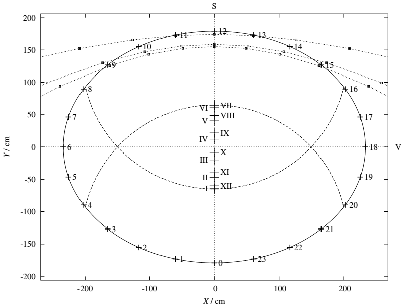
Obr. 6 — Schéma analematických hodin v Bohdanči, spočtené programem SHA. Hodinové značky na schématu jsou popsány arabskými číslicemi, datová úsečka římskými, čárkované čáry znázorňují části Lambertových kružnic pro letní a zimní slunovrat. Tečkované křivky se čtveřky přibližně značí, kam dosahuje stín člověka (ukazatele) vysokého 180 cm v různých denních a ročních dobách.
